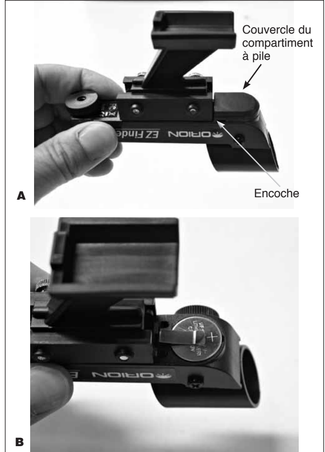
Figure 10. A) Pour installer la pile CR2032 dans l'EZ Finder II, tournez-la à l'envers puis retirez le couvercle du compartiment à pile. B) Installez la pile avec le pôle positif (+) vers le haut, comme illustré.
