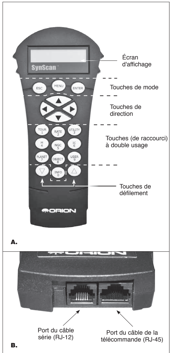
Figure 17. A) La télécommande GoTo SynScan V4, B) Port du câble de la télécommande et port du câble série sur la base de la télécommande.
