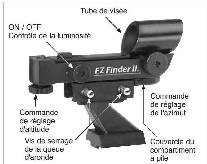
Figure 11. Bouton ON / OFF (Marche / arrêt) et boutons de réglage de l'EZ Finder II
