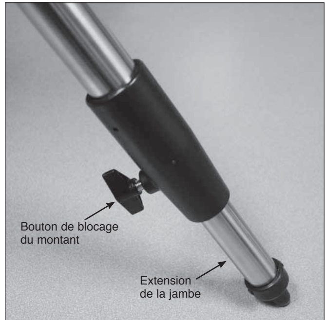
Figure 6. Desserrez le bouton de serrage du montant pour ajuster la longueur des montants du trépied.
