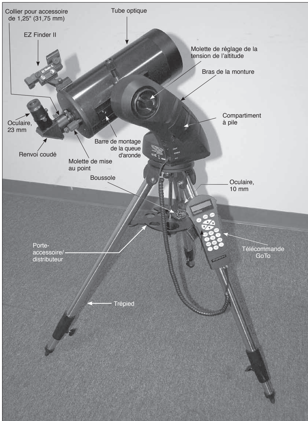
Figure 1. Pièces du StarSeeker IV (Maksutov-Cassegrain 127 mm illustré)
