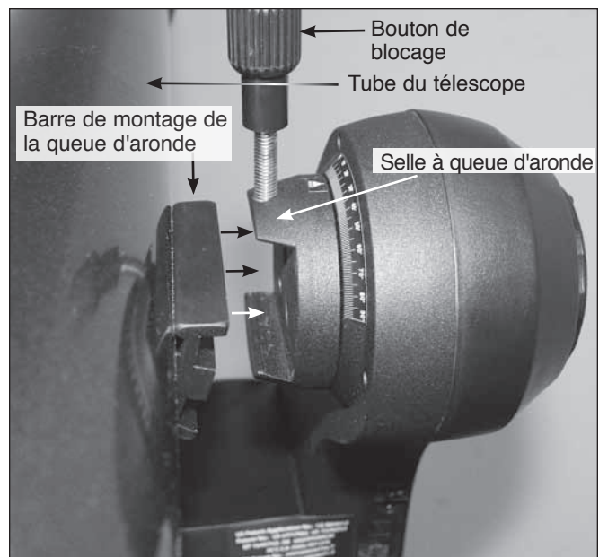
Figure 7. Le tube du télescope peut être attaché et retiré facilement via la selle en queue d'aronde sur le bras de la monture.
